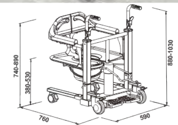
YJL-8950 液压式移位机
