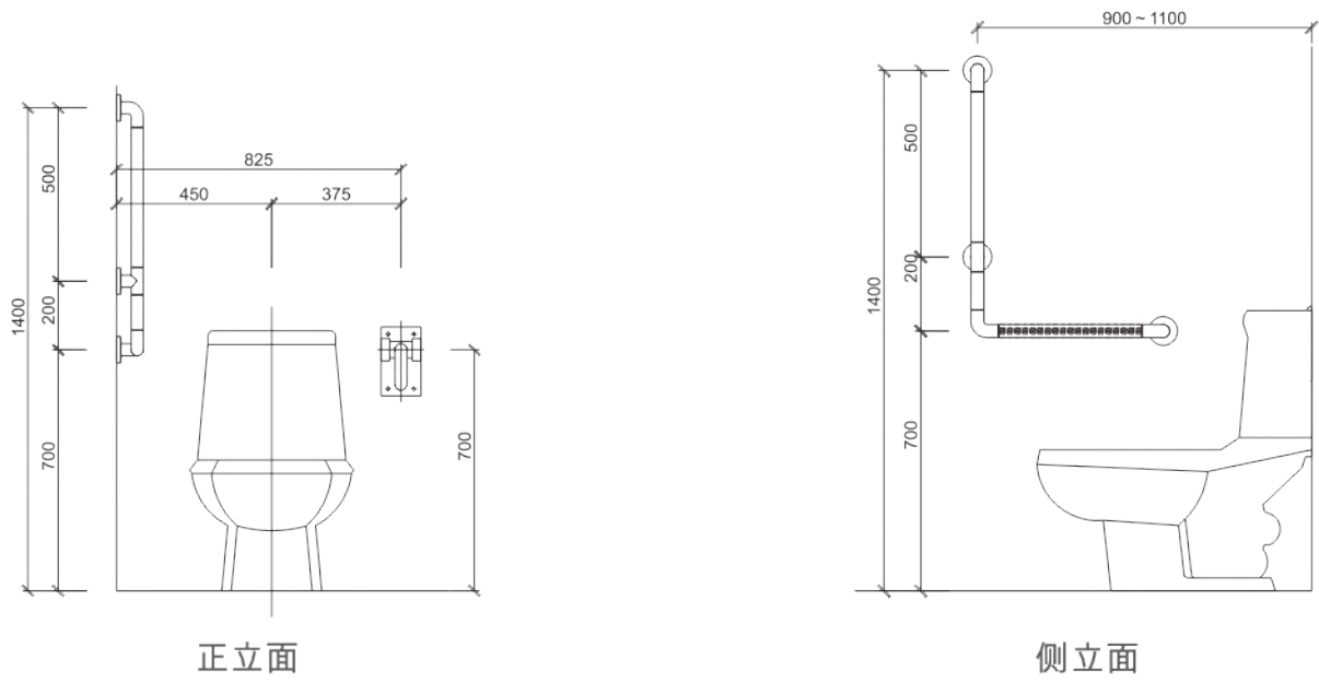
成人无障碍安装图
